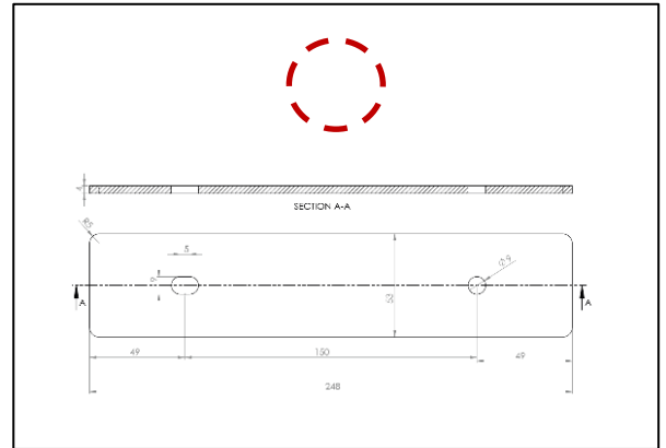
Samlebeslag varenr: 26381
