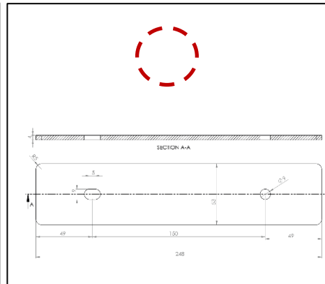
Samlebeslag varenr: 26381
